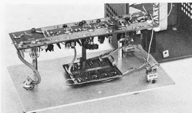
Beim Internationalen Bodenseetreffen des DARC in Konstanz fand dieser 2-m-Fuchsjaagd-Sender viel Beachtung. Er ist mit einem Zeichengeber sowie integrierten Schaltungen bestückt und arbeitet mit tonloser oder tönender Telegrafie (Aufnahme: DJ 8 PO)
