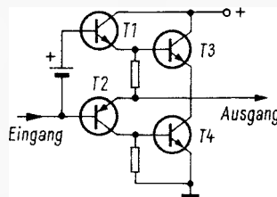
Bild 1. Prinzip der quasi-komplementären Endstufe
