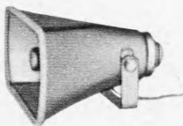
SC-15B Abmessungen 387 x 207 mm Leistung 15 Watt Widerstand 8 Ohm
