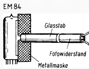
Bild 2. Die Anordnung des Fotowiderstandes 7412 (RCA) im Rohr, Lichtführungsstab, Metallmasken und Röhre EM 84
