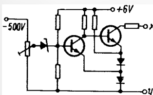
Bild 3. Der elektronische Schalter
