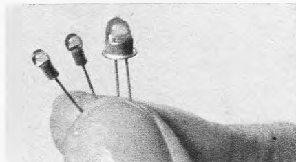
Links zwei der neuen Miniatur-Leuchtelemente mit sehr kleinem Halter (2,5 mm \phi ) im Vergleich zu konventionellen Elementen. Sie eignen sich als Signallampen in Geräten, für optoelektronische Anwendungen und für alpha-numerische Darstellungen an Digitalrechnern
