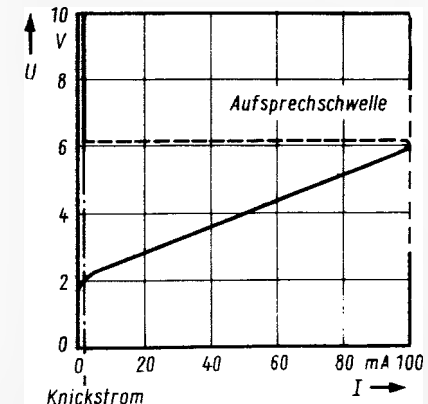
Bild 2. Spannungs-Strom-Kennlinie der Sicherung
