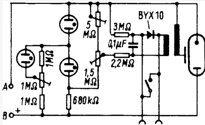
Bild 5. Schaltung des Lampenstabes
