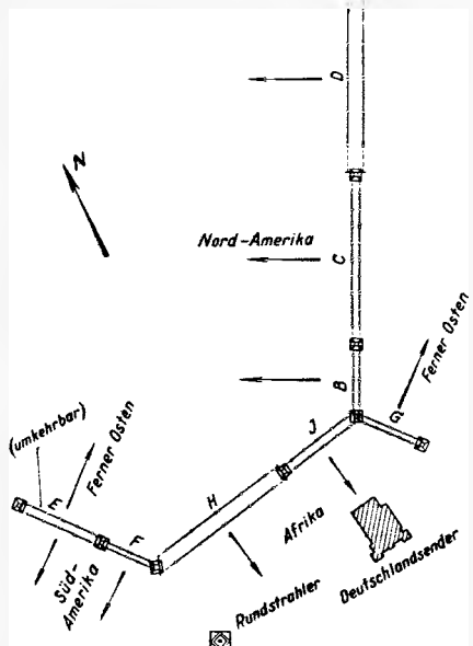
Bild 5. Antennenanlage des deutschen Weltrundfunksenders Zeesen. Ende 1932 gab es nur den Rundstrahler und die Tannenbaum-Richtstrahlantennen B, C und D für die Senderichtung Nordamerika. Die Antennen E bis J wurden am 1. 2. 1934 in Betrieb genommen
