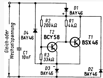
Bild 1. Schaltung der bipolaren Überstromsicherung (nach Siemens-Halbleiter-Schaltbeispiele 1969)
