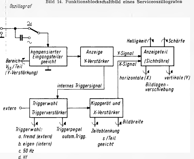
Bild 14. Funktionsblattschaltbild eines Serviceoszillografen
