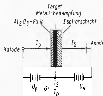
Bild 1. Meßschaltung zur Ermittlung der Ausbeute von Sekundärelektronen nach dem Durchschußprinzip
