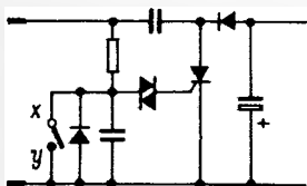
Bild 2. Triggerung des Thyristors durch einen Diac
