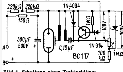
Bild 6. Schaltung eines Tochterblitzes
