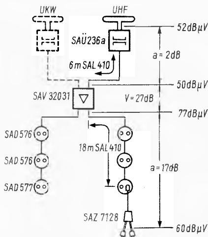
Bild 1. Pegelrechnung im UHF-Bereich, durchgeführt am Beispiel einer kleinen Gemeinschaftsantennen-Anlage mit Mehrbereichsverstärkern. Im UKW-Bereich kann selbstverständlich analog vorgegangen werden
