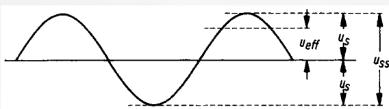
Bild 12. Darstellung und Zusammenhang zwischen u_{eff} , u_s - und u_{SS} -Werten einer Sinusspannung
