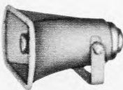
SC-10B Abmessungen 301 x 179 mm Leistung 10 Watt Widerstand 8 Ohm
