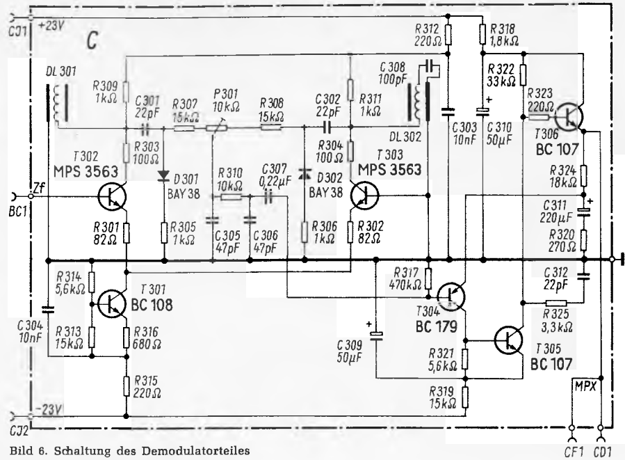
Bild 6. Schaltung des Demodulatorerteiles
