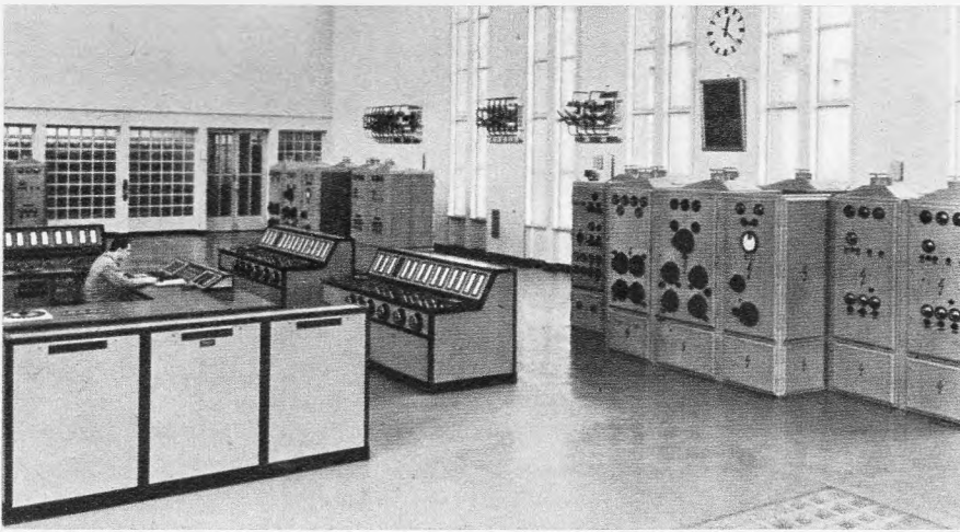
Bild 4. Senderhaus 4 in Zeesen mit vier 50-kW-„Olympia“-Sendern von Telefunken ab Juli 1936. Jeder Sender hatte sieben Stufen und war mit zwei je 25 kW leistenden Endstufen ausgestattet. Eine 25-kW-Endstufe enthielt 2 \times 2 RS 257 parallel und in Gegentakt; beide Endstufen wurden von der gemeinsamen fünften Stufe ( 2 \times RS 207) angesteuert
