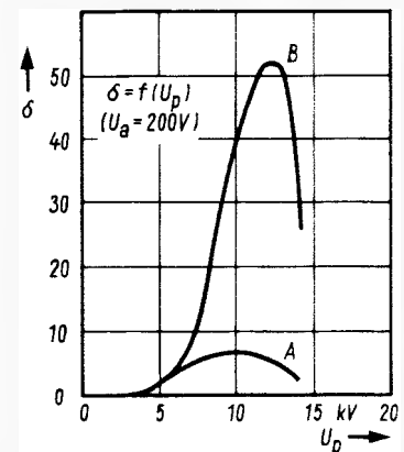
Bild 2. Sekundärelektronenausbeute \delta bei homogener (A) und porösem Material (B)
